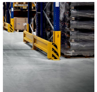
Rammschutz zur Vermeidung von Anfahrsschäden, z. B. in Eck-bereichen oder an Regalstützen.
