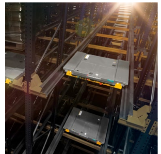
Das Jungheinrich UPC unterfährt die Paletten und ist flexibel anpassbar an Ihr Einsatzszenario.
