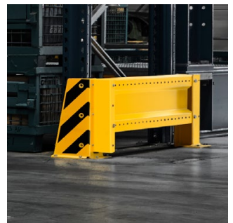
Um die Regale vor einer Kollision mit Flurförderzeugen zu schützen, kommen Flurförderzeugabweiser als Rammschutz zum Einsatz.
