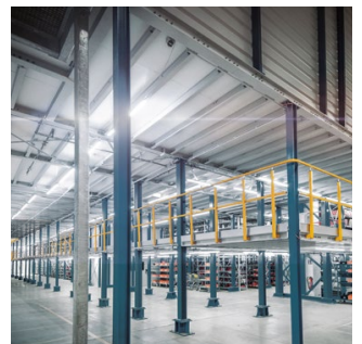
Die selbsttragende, begehbare und optional befahrbare Konstruktion der Stahlbaubühne schafft auf mehreren Geschossen zusätzliche Fläche.
