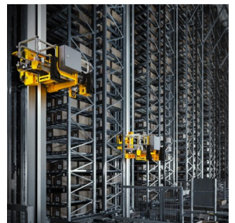
Automatische Kleinteilelager sind die erste Wahl in Hochleistungsumgebungen wie z. B. Ersatzteillagern oder Distributionszentren.
