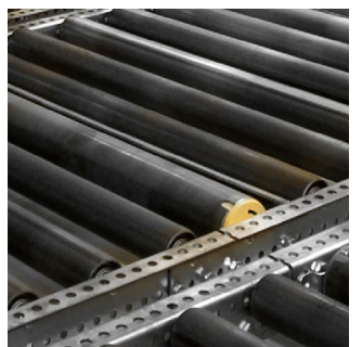
Beim Durchlaufregal kontrollieren Bremsrollen das Tempo des Palettentransports.
